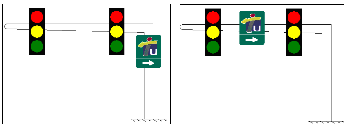
Figura 34. Ejemplos de instalación del rótulo TU adherido a un poste o brazo del sistema de semáforos.
