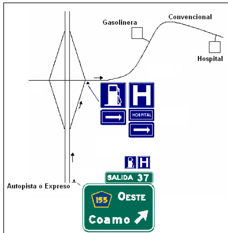
Figura 22. Ejemplo de instalación de rótulos de servicios generales al conductor como placas auxiliares en un rótulo de orientación de destino.
