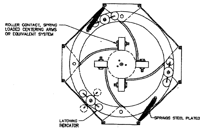
TOP VIEW MOUNTING RING SCALE: N.T.S.
