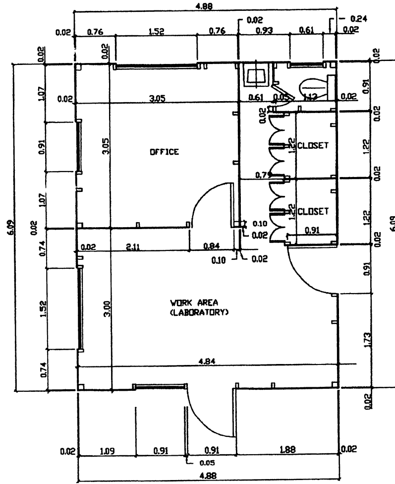
PLAN SCALE: 1/32
